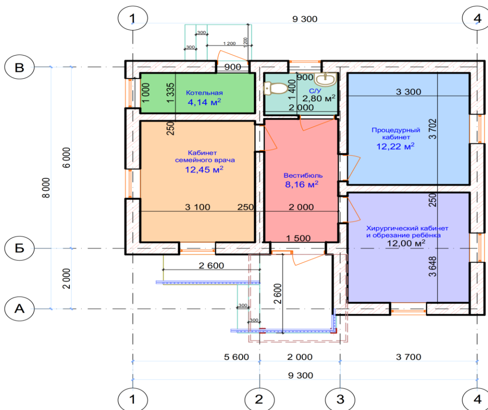
Предварительный план медицинского пункта в селе Вишхарв
