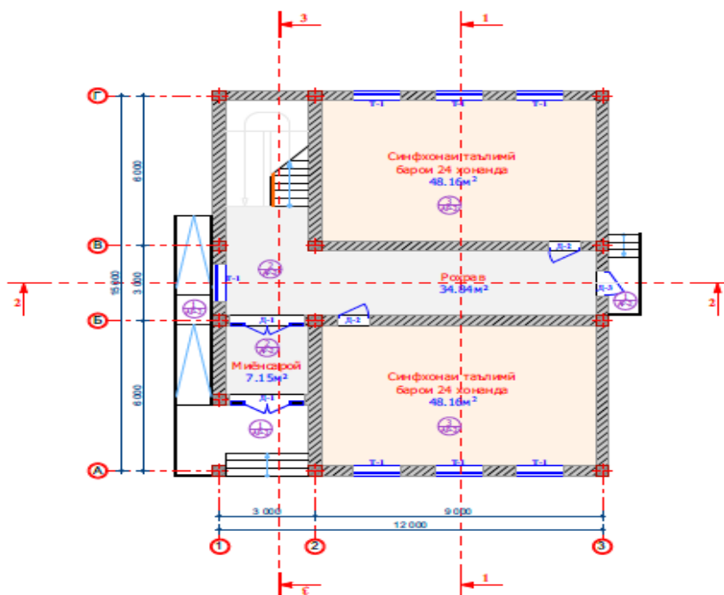
План 1-го этажа средней школ в селе Правда
