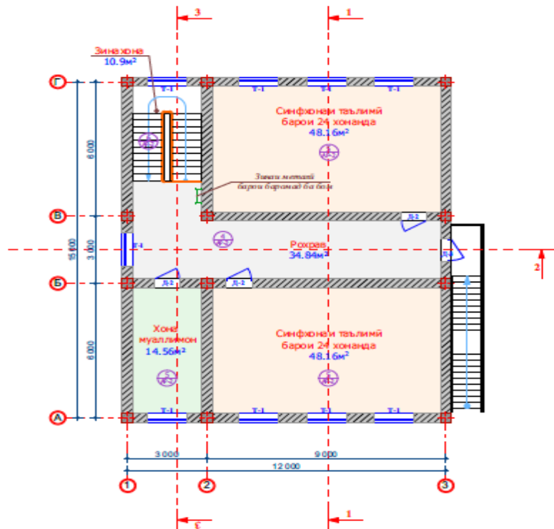
План 2-го этажа средней школ в селе 15-Таджикистан
