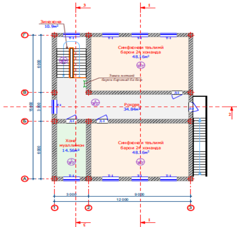
План 2-го этажа средней школ в селе Навобод
